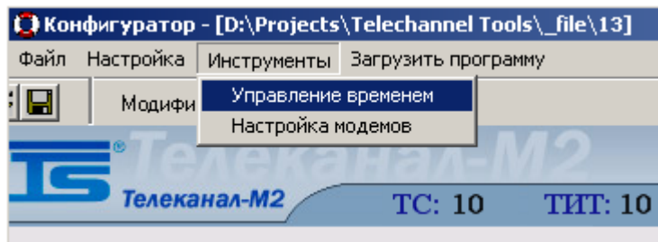
Рисунок 22 – Меню «Инструменты».
